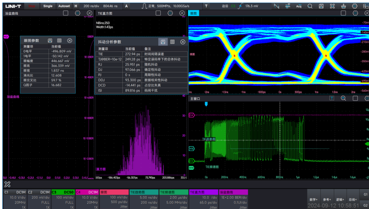
抖动分析和眼图选件具备完备的抖动测量算法以及丰富的抖动分析视图
