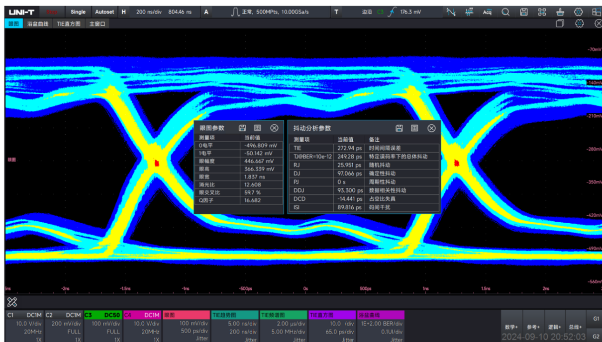
对 USB2.0 标准协议信号进行眼图分析，并测量其眼图相关参数
