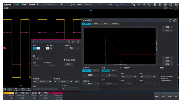
用户自定义的高级滤波设计器，在示波器即可完成
