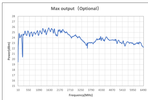
最大输出功率实测值
