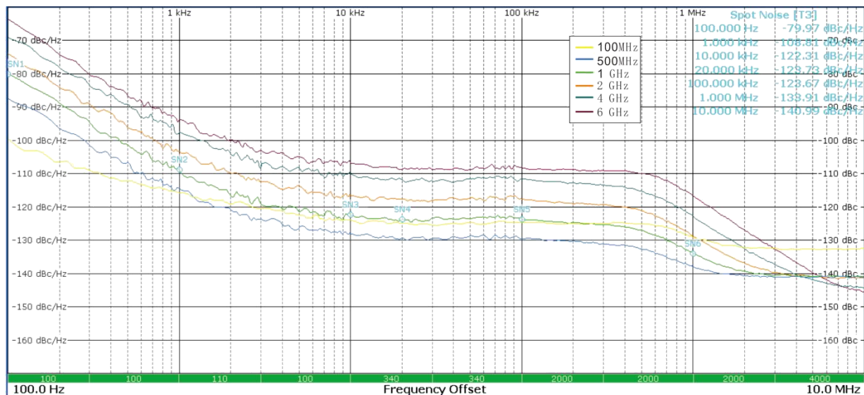
单边带相位噪声实测值
