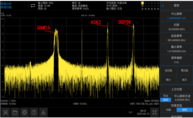
不同调制类型多载波实测图
