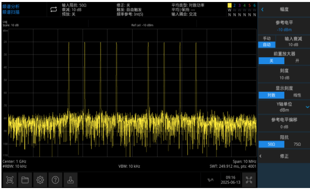
多音调制实测频谱图
